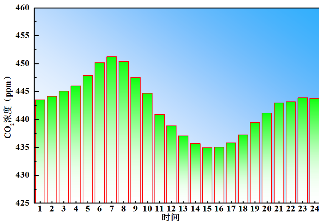
图 2 大气 CO 2 逐时平均浓度变化
