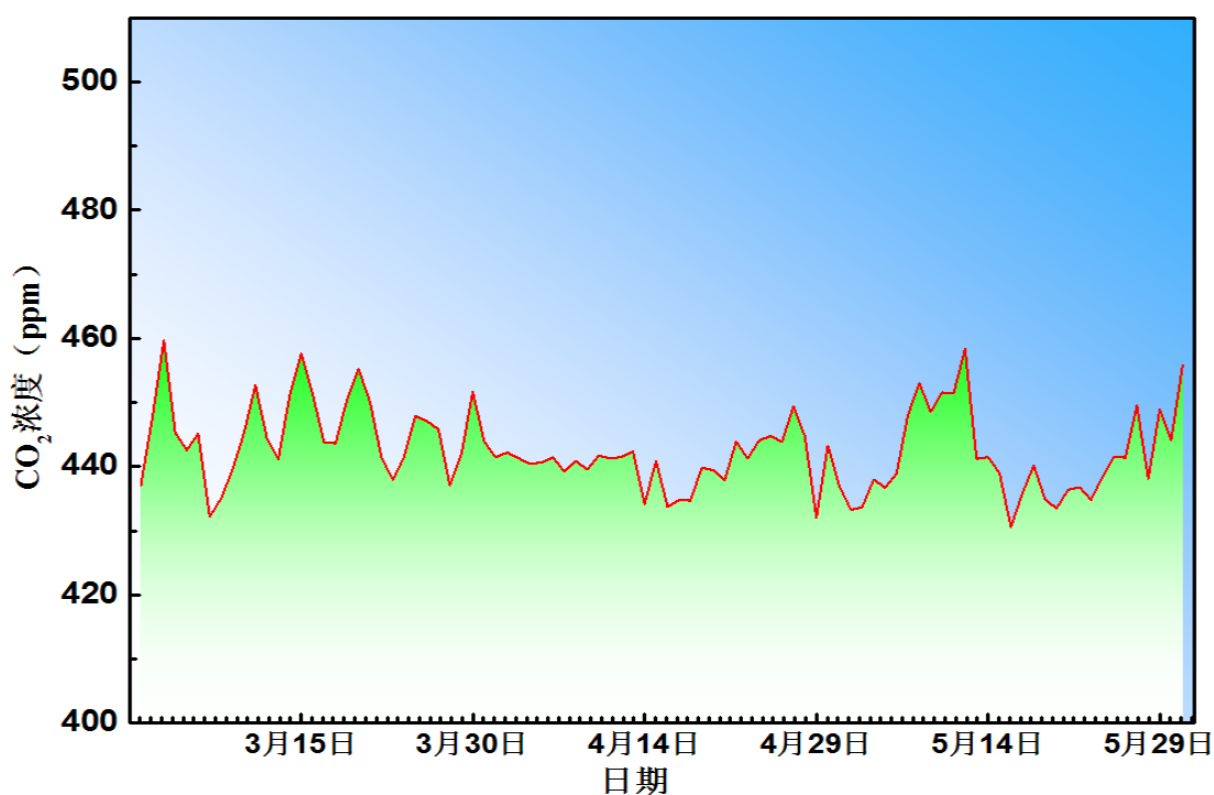
图 3 大气 CO 2 逐日浓度变化
