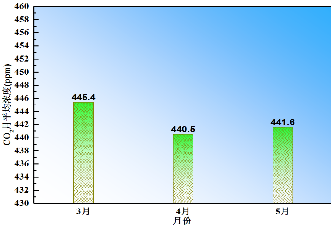
图1 大气 CO 2 月均浓度变化
