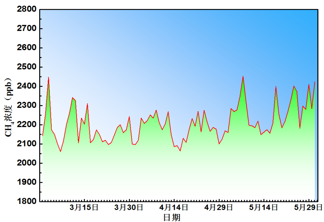
图6 大气 \text{CH}_4 逐日浓度变化
