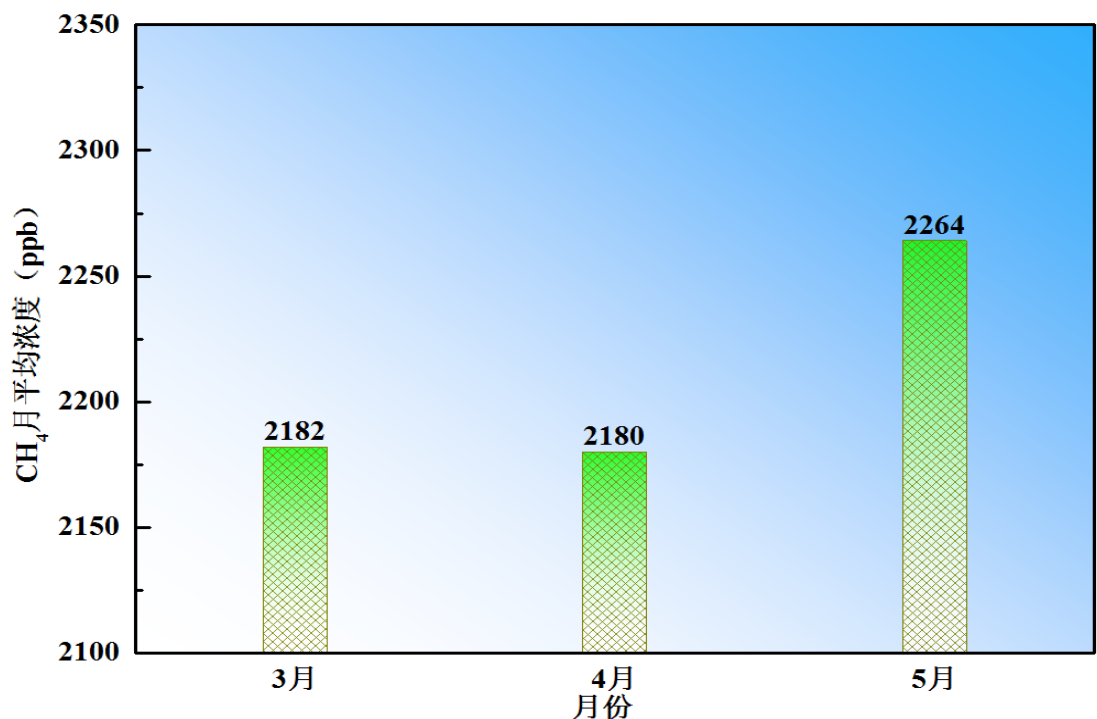
图4 大气CH 4 月均浓度变化
