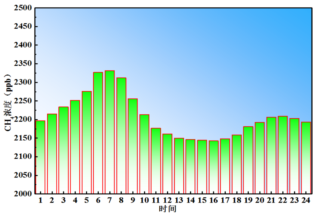
图5 大气 \text{CH}_4 逐时平均浓度变化
